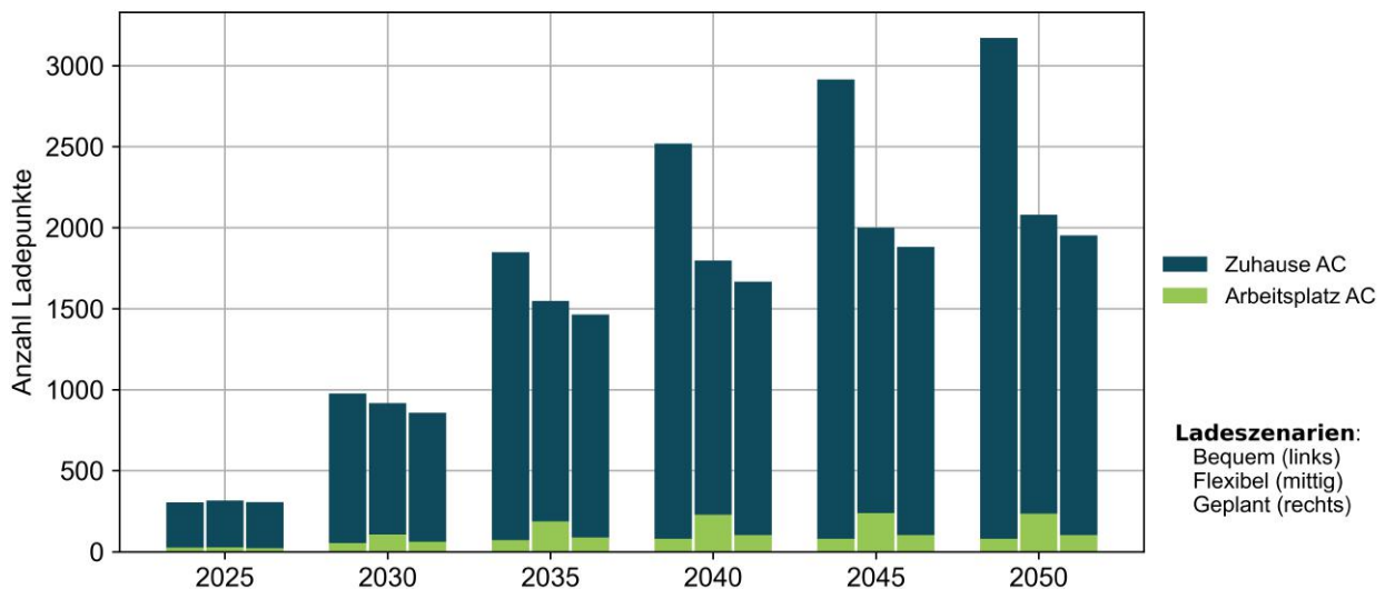
Szenarien für private Ladepunkte: Gemeinde Diepoldsau. [3]
