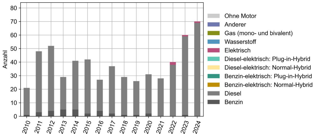
Anzahl der Inverkehrsetzungen im Sachtransport nach Antriebsart: Gemeinde Diepoldsau. [8]
