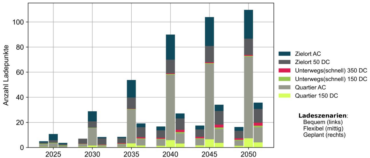
Szenarien für allgemein zugängliche Ladepunkte: Gemeinde Diepoldsau. [3]
